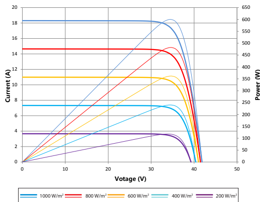
电流-电压 & 功率-电压曲线图 (600S)
