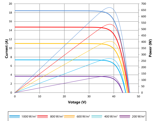
电流-电压 & 功率-电压曲线图 (670S)
