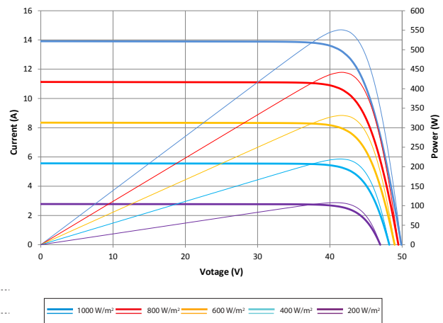
电流-电压 & 功率-电压曲线图 (550S)
