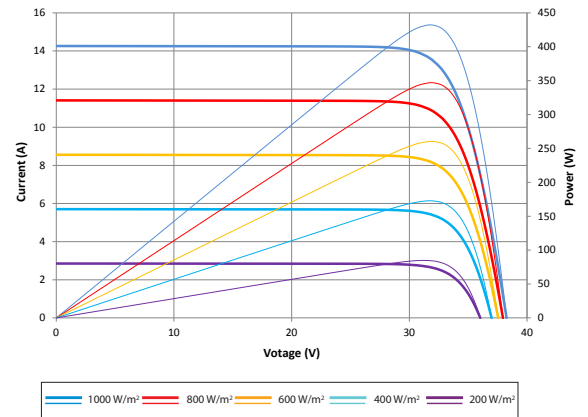
电流-电压 & 功率-电压曲线图 (430S)
