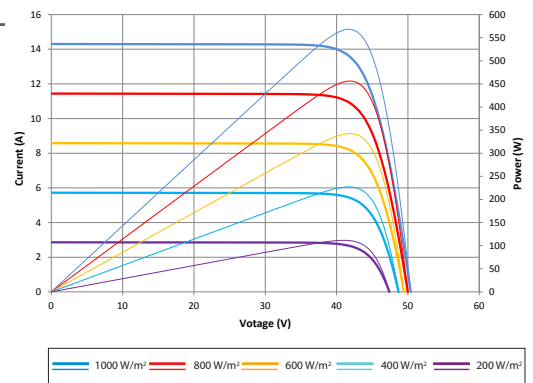
电流-电压 & 功率-电压曲线图 (570S)
